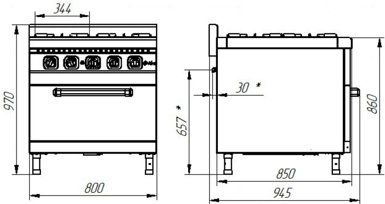
Габаритные размеры газовой плиты ПГК-49ЖШ-II-A
