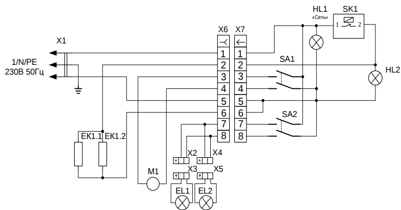
Схема электрическая принципиальная ШРТ 10М
