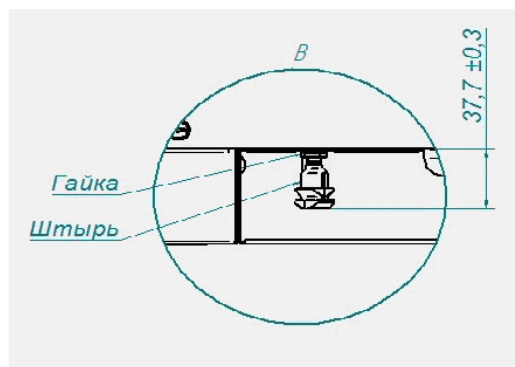
Вид сверху
