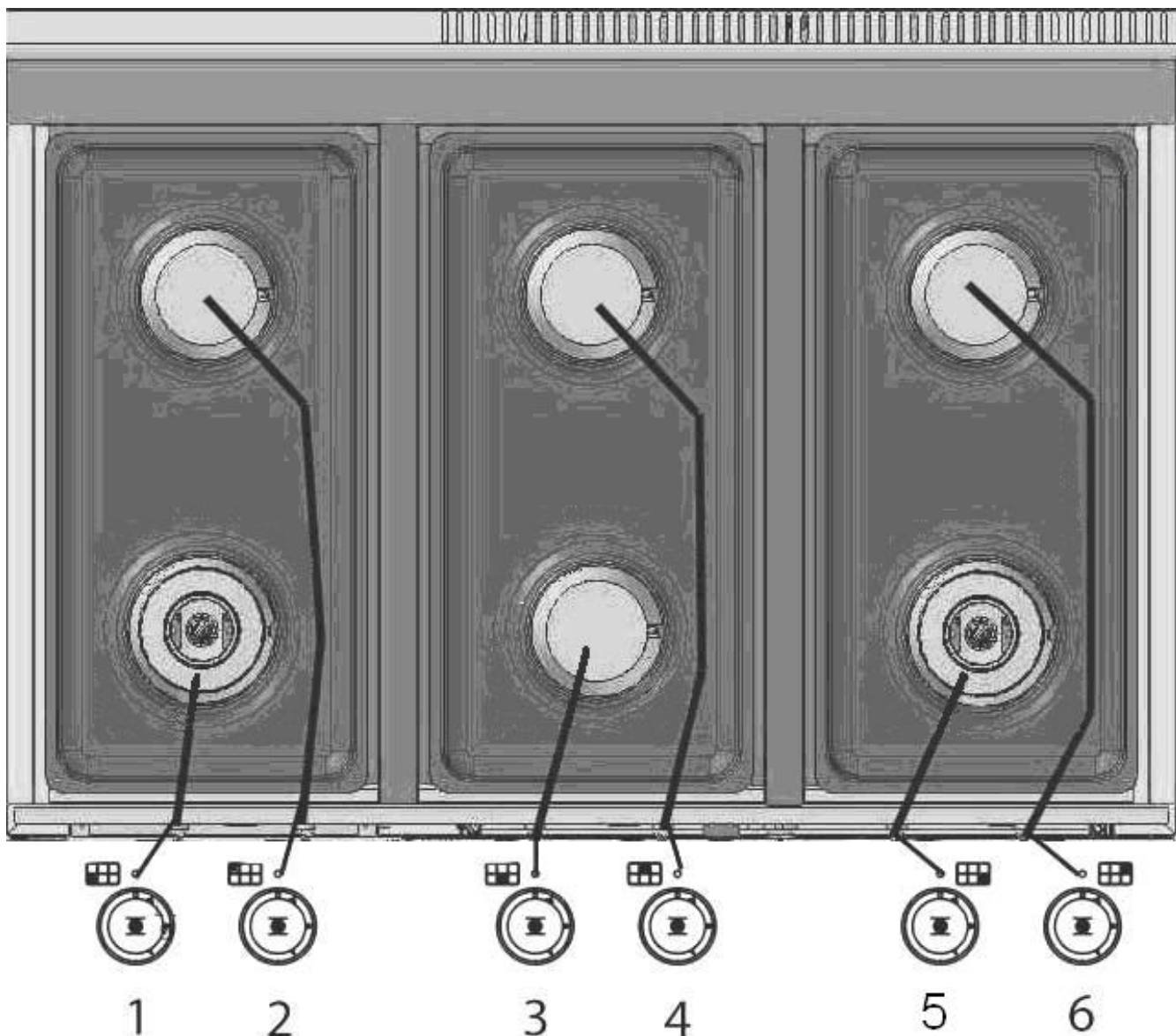
Рис. 4 Плита ПГК-69П-II-A
