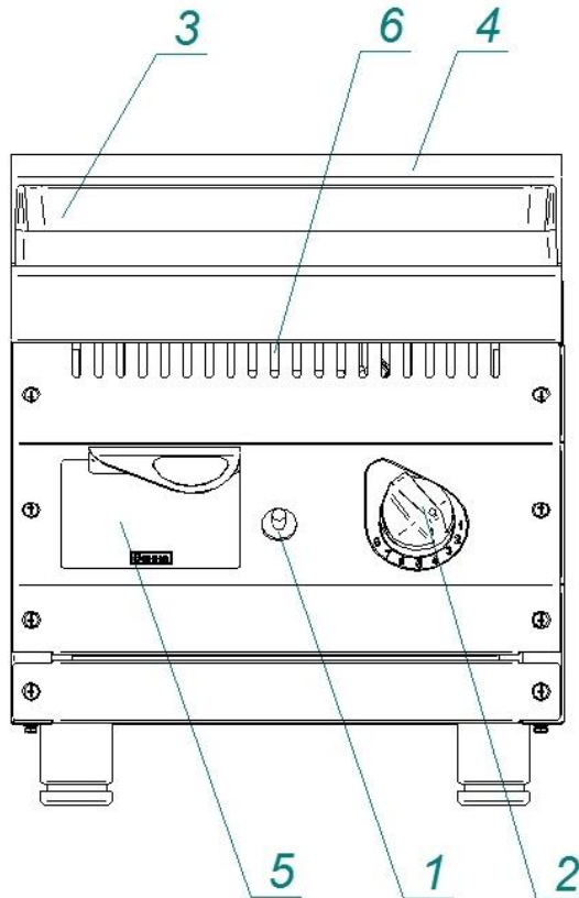
Рис. 1. Аппарат газовый
